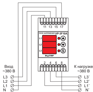
Схема подключения
