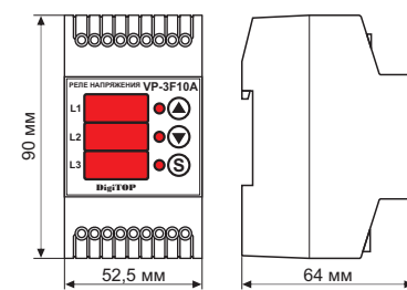
Габаритные размеры
