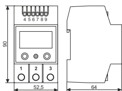
Габаритні розміри
