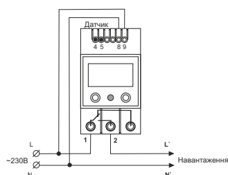
Схема підключення
