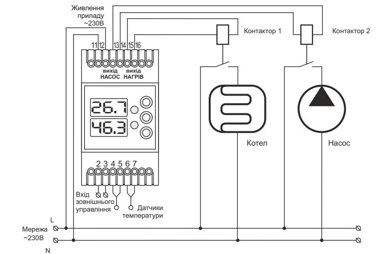
Призначення виводів
