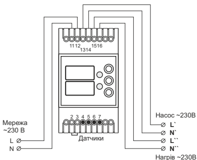
Схема підключення
