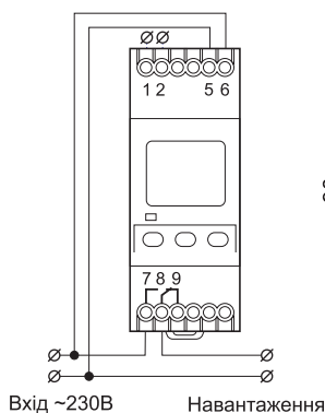
Схема підключення
