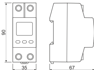
Габаритні розміри
