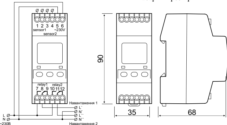
Схема підключення
